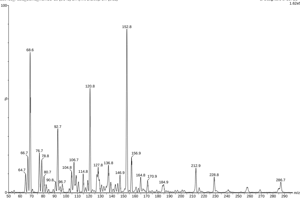
Fig. 7: Kaempferol.
