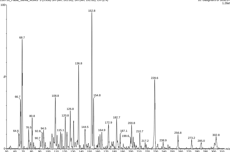
Fig. 8: Quercetin
